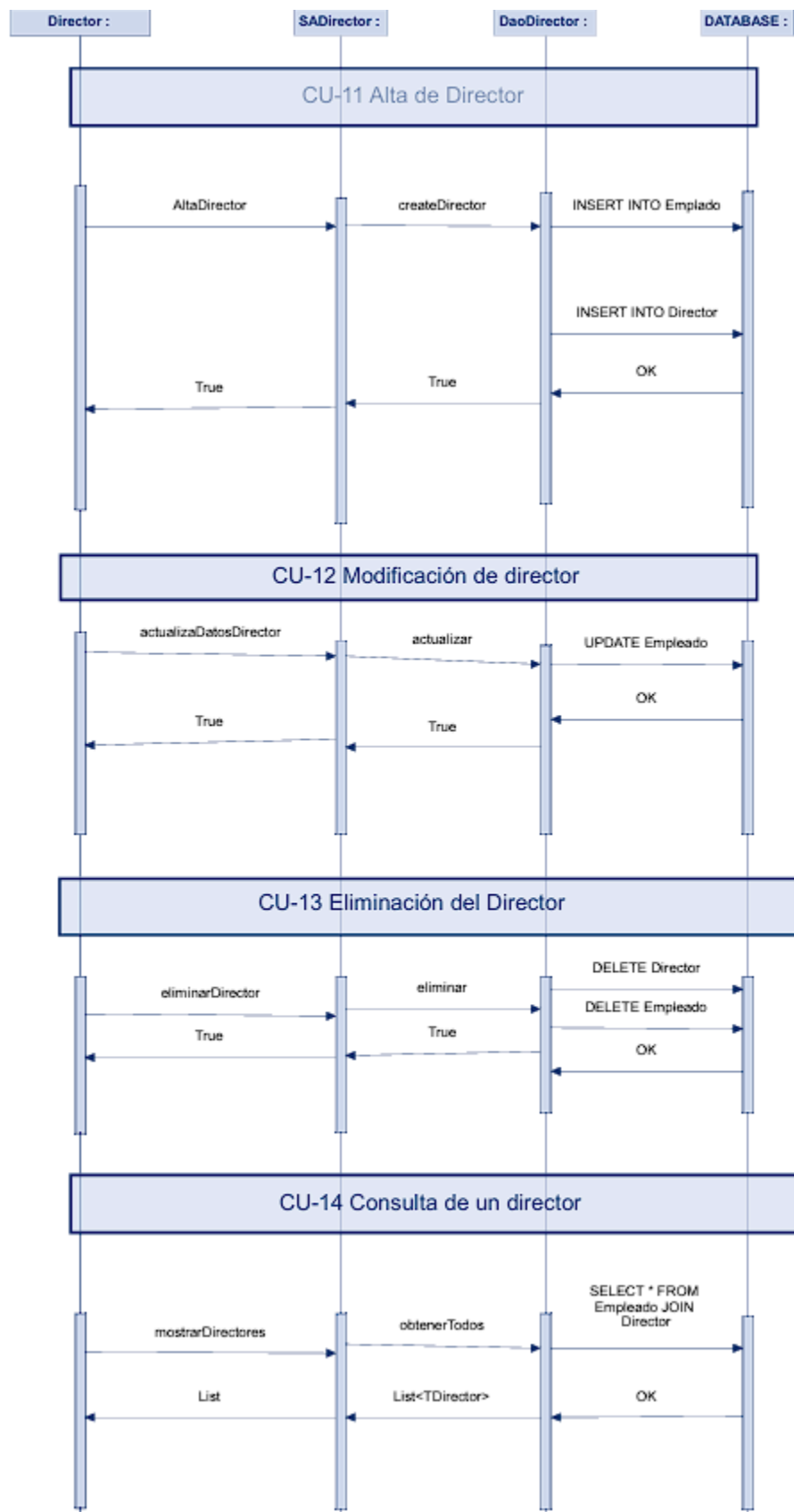
Figura 7-10. Diagrama de secuencia de Directores
