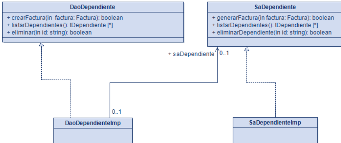
Figura 7-7. Diagrama de clases de Dependientes
