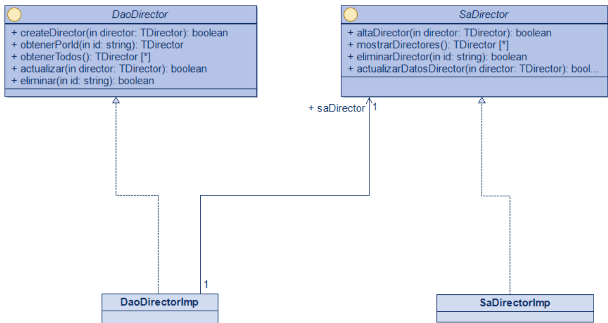
Figura 7-9. Diagrama de clases de Directores
