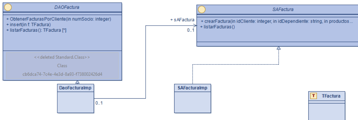
Figura 7-3. Diagrama de clases de Facturas
