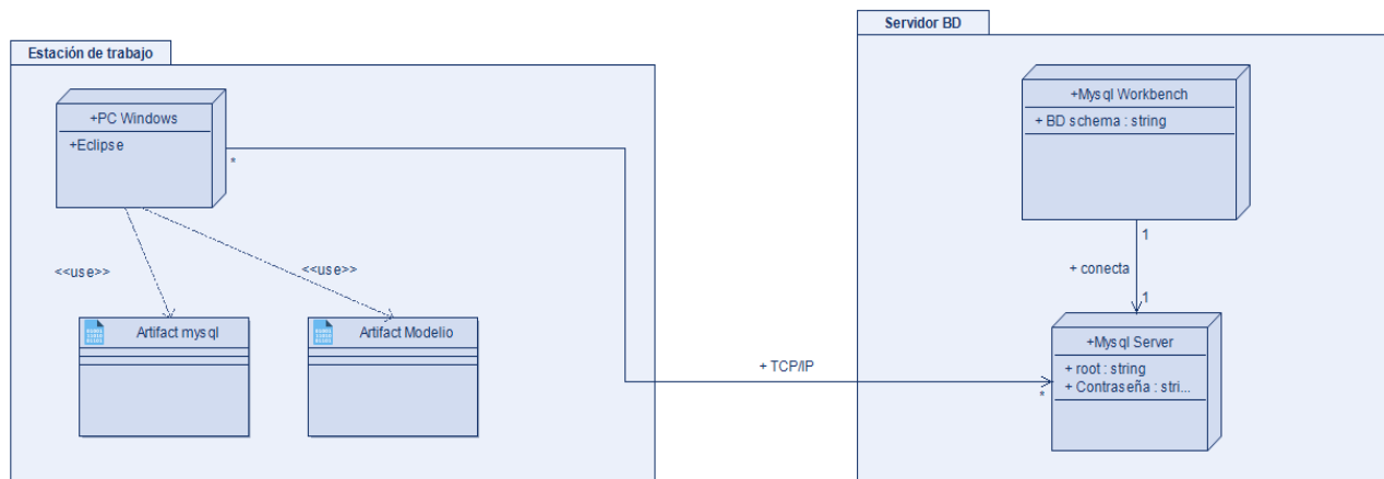
Figura 7-1. Diagrama de despliegue
