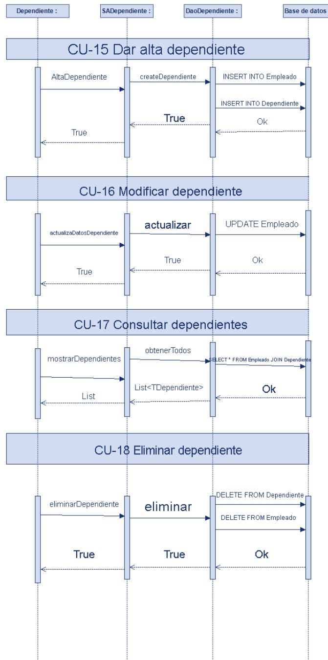
Figura 7-8. Diagrama de secuencia de Dependientes
